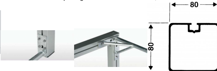
Haspo Jugendtor Kleinfeldtor 1201, 1401
