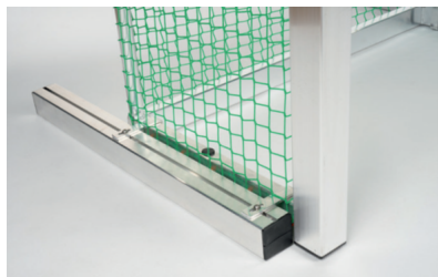
Haspo Zusatzgewicht für Minitor FTZH01350
