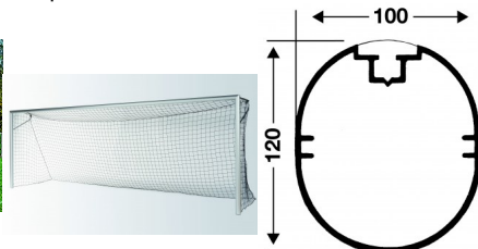
Haspo Großfeldtor in Bodenhülsen 100
