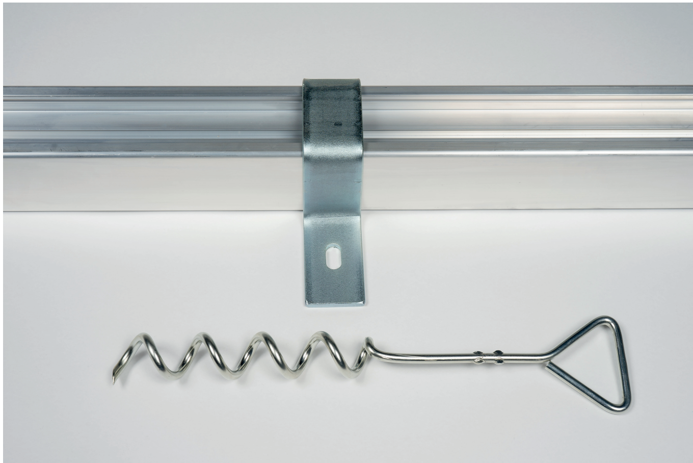
Haspo Sicherheits-Verankerung für Fußballtore Standard 122219
