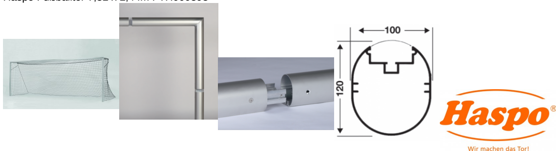
Haspo Fußballtor 7,32 x 2,44m FTH000898
