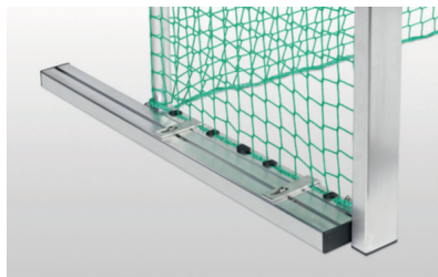
Haspo Zusatzgewicht für Minitor FTZH01340
