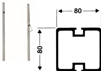
Multi-Spielpfosten VBH000541
