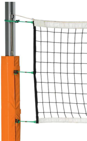
Haspo Säulenschutzpolster 5172
